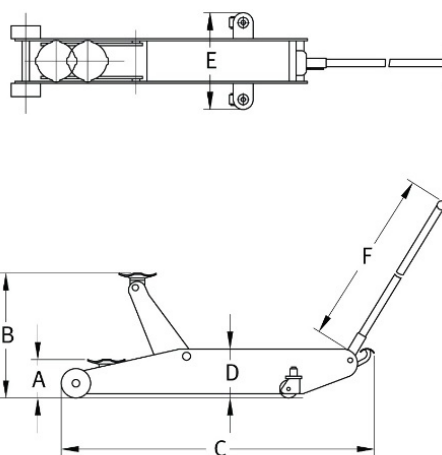
Desenho dimensional
